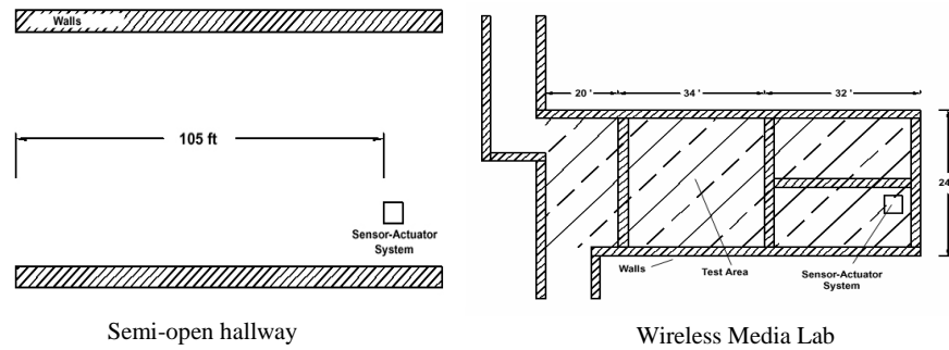
Fig. 9. System Test Scenarios
